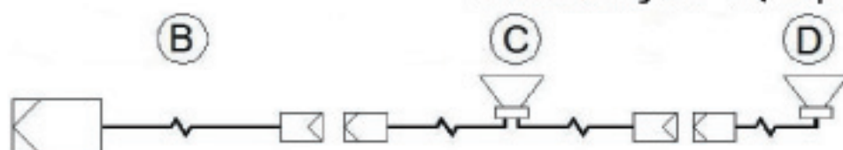
AA Bekabeling voor 4+ (=2 speakers)
